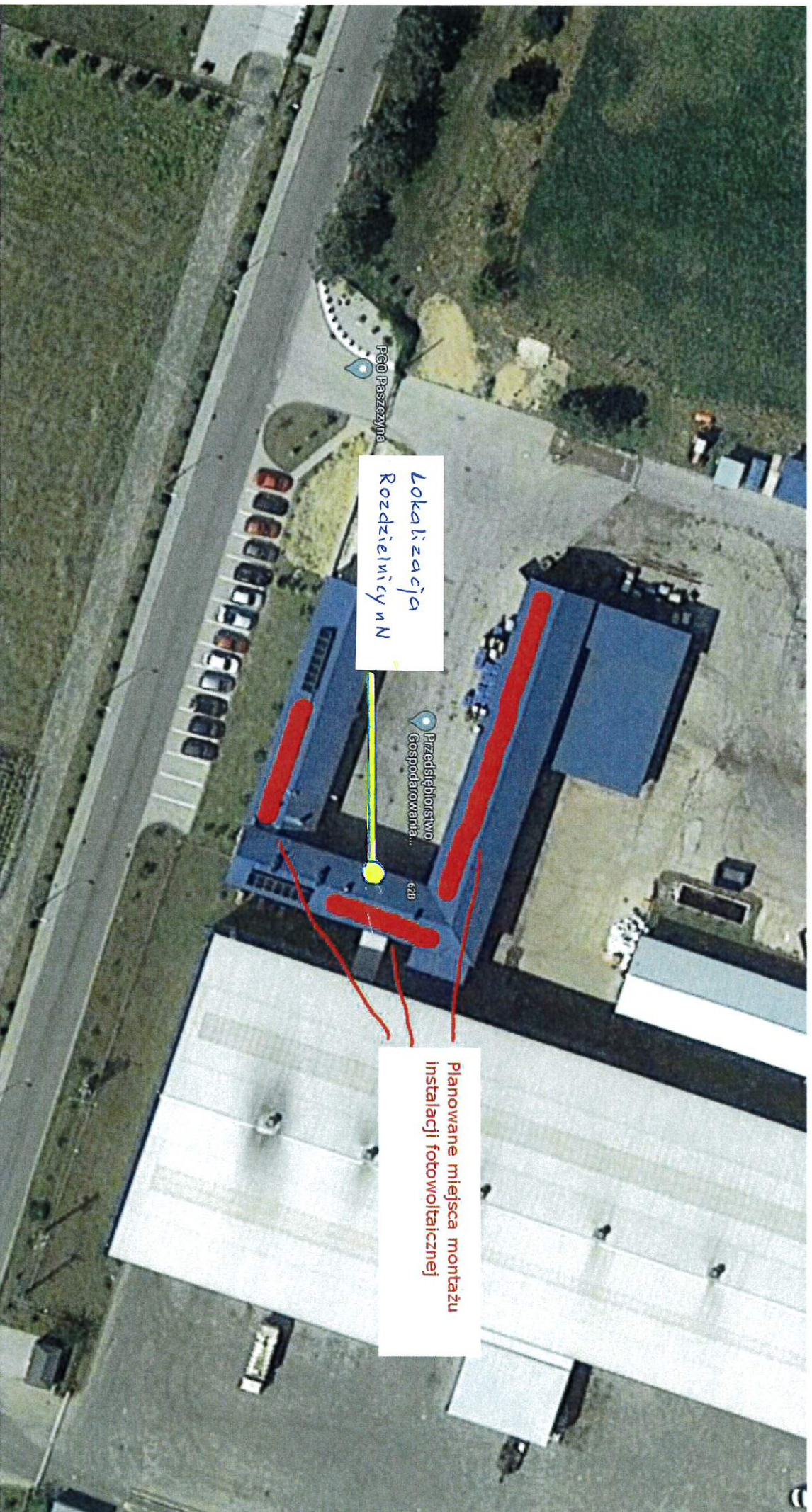
Lokalizacja rozdzielniczy nN, w którą ma być wpięta instalacja fotowoltaiczna.
